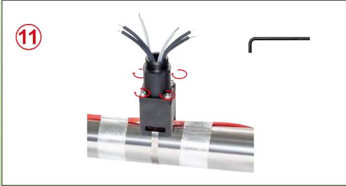
11: 用4个螺丝将脚的上部拧紧，直到两个配件接触，从而压缩密封件
