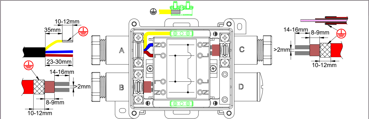
带2根发热线和一根电源电缆的型号 (YB13)
