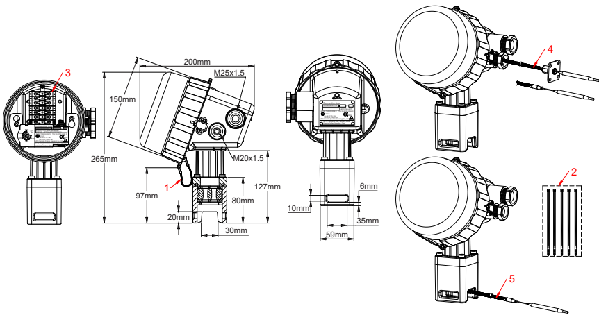
1: 盖子链条, 2: 红色扎带, 3: 接线柱套件, 4: 通过M20电缆接头的毛细管输出, 5: 通过管道安装脚的毛细管输出。
