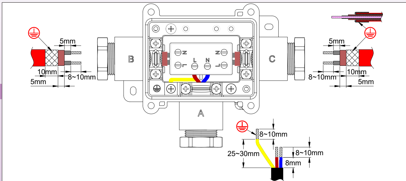
带2根发热线和一根电源电缆的型号 (YC3)
